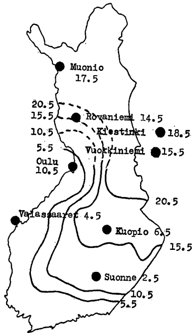
Kartta 2. Keskimääräinen jäidenlähtöaika Suomessa vuosina 1892–1931 SIMOJON mukaan. Karttaan on merkitty kuikan saapumisaika eräille paikkakunnille pistein. Havainnoitsijat eri paikkakunnilla ovat: Muonio (Montell), Rovaniemi (Komonen), Kiestinki – Röhö (Lampio ja Lehtonen), Vuokkiniemi – Luomajärvi (Lampio ja Lehtonen), Oulu (Merikallio), Kuopio (E. V. Suomalainen), Valassaaret (Hildén) ja Suonne (Lehtonen).
